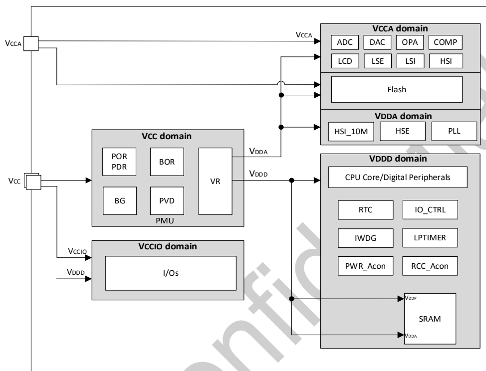
图 2-2 电源框图
