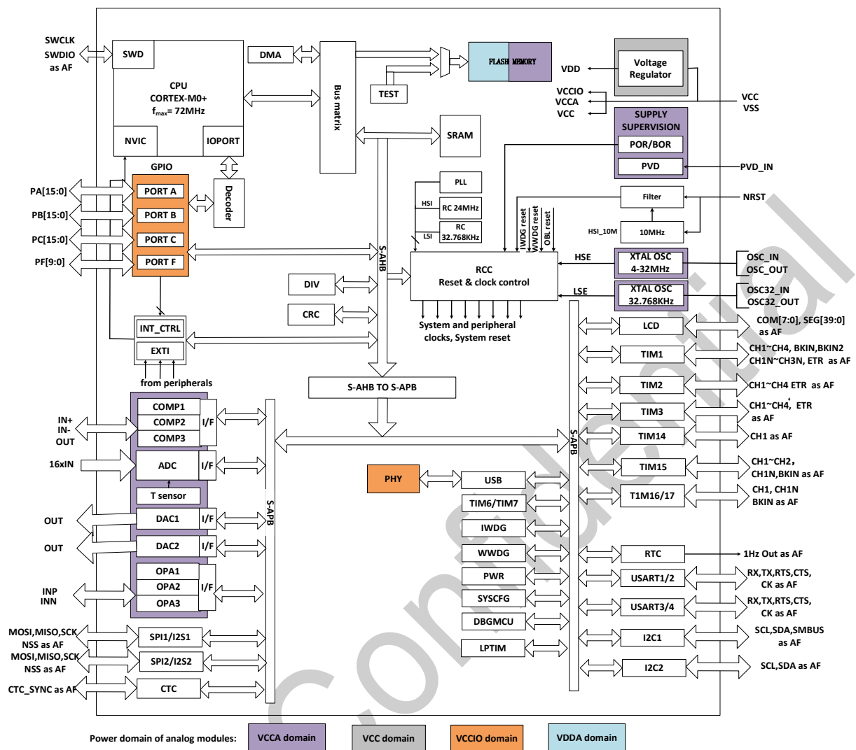
图 1-1 功能模块
